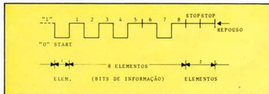
Figura 7 — Estrutura de um caráter Assíncrono
